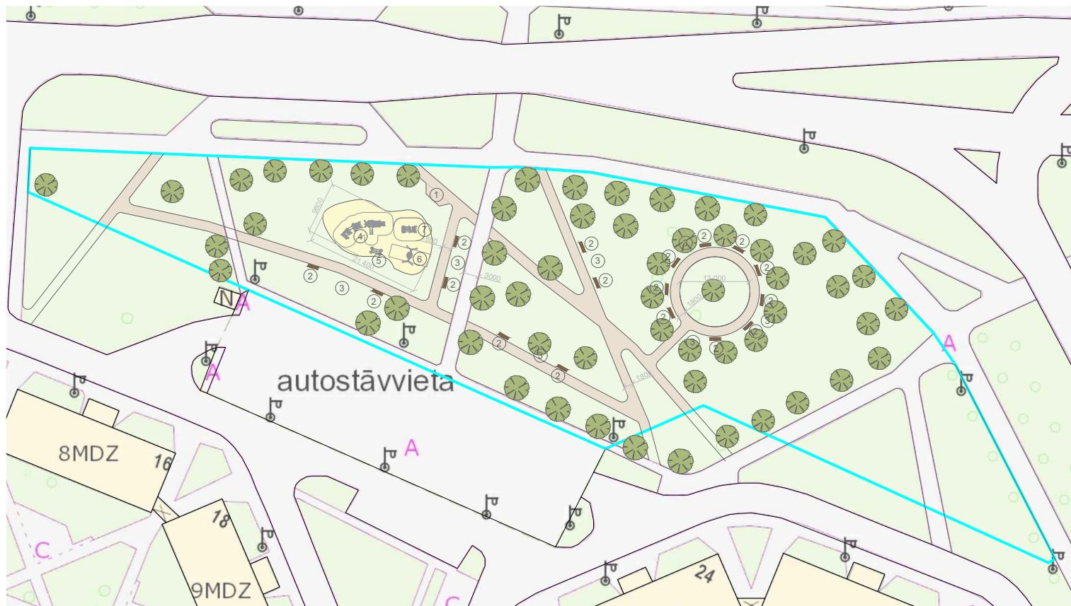
ĢENERĀLPLĀNS, M 1:1000
