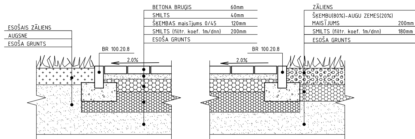
GĀJĒJU UN VELOSIPĒDU CEĻA PRINCIPIĀLS ŠĶĒRSGRIEZUMS
